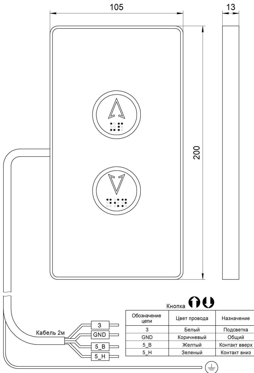
Рис.1 Внешний вид, габаритные и установочные размеры Вызывного поста МАЛАХИТ НШЕК.468381.063
